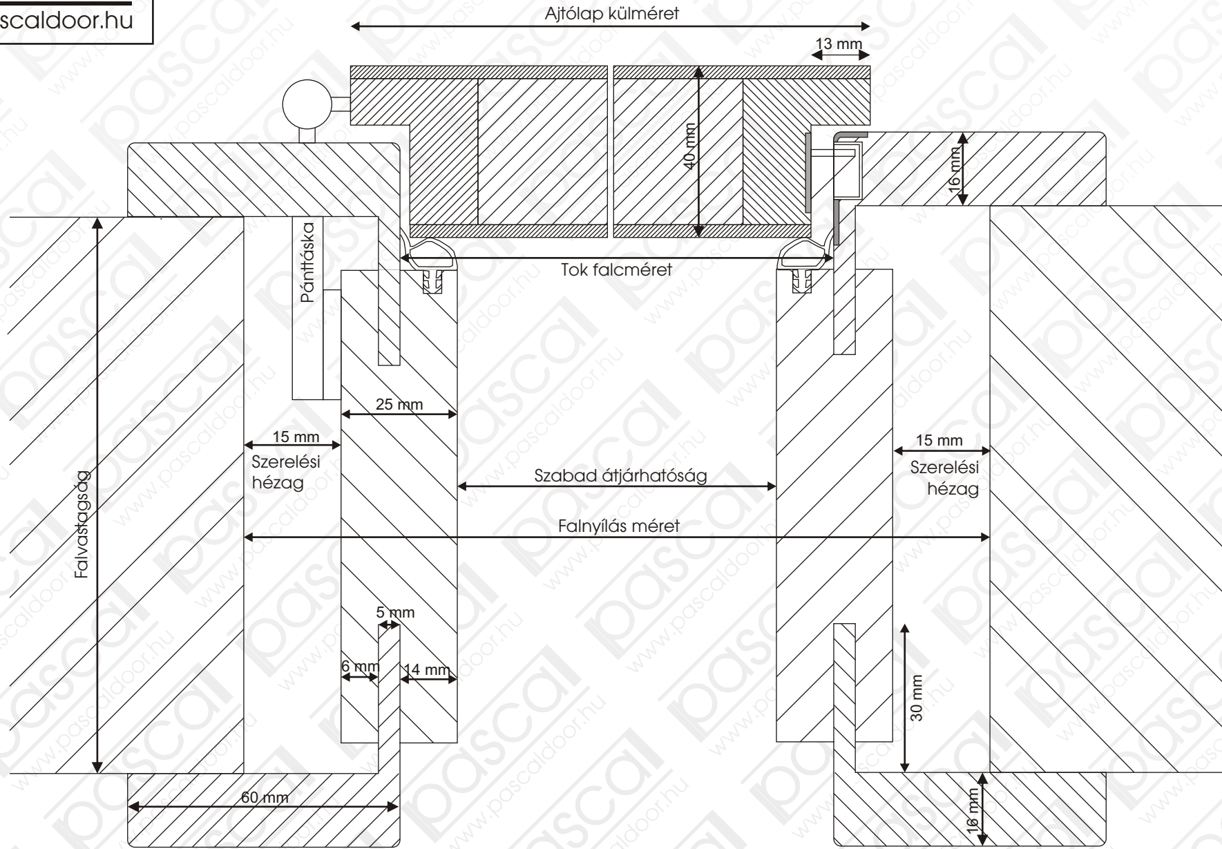
PASCAL ajtó vízszintes tokmetszet
